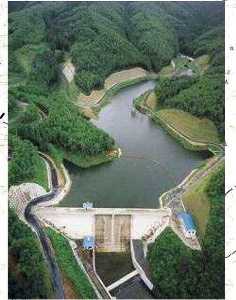
千松ダム
